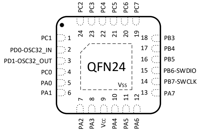
图 3-1 QFN24 Pinout1 PY32CA80E16U7
