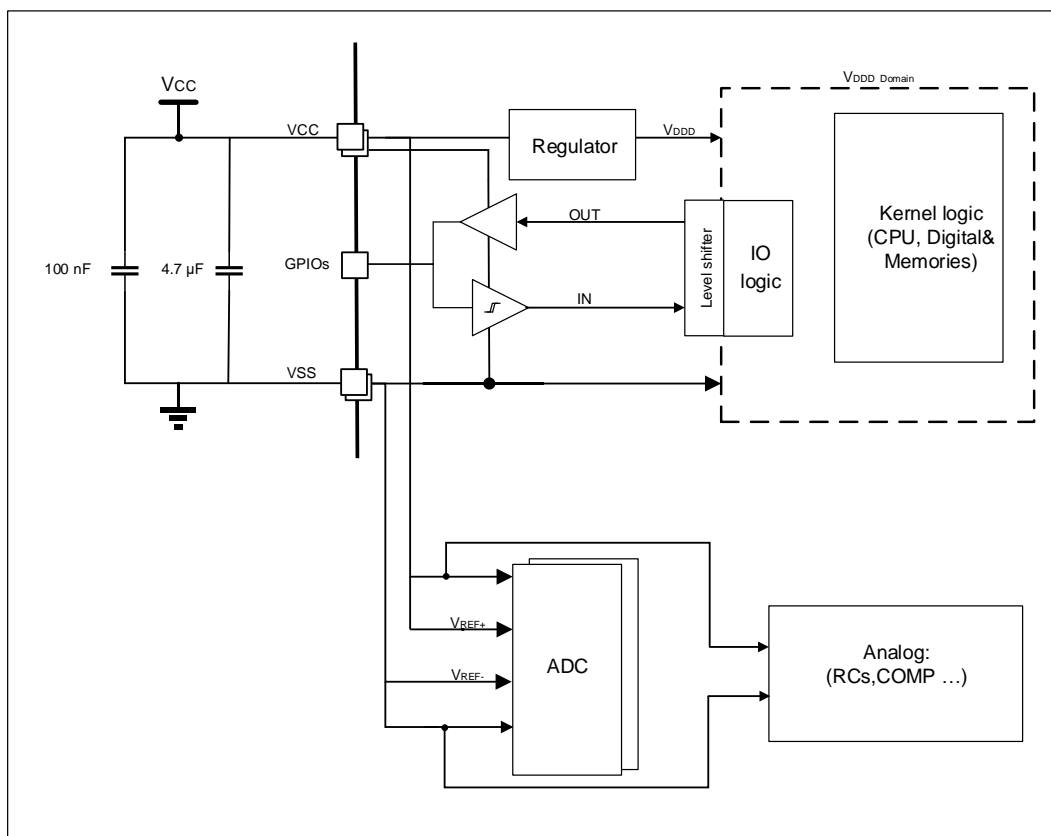
图 5-1 供电方案图
