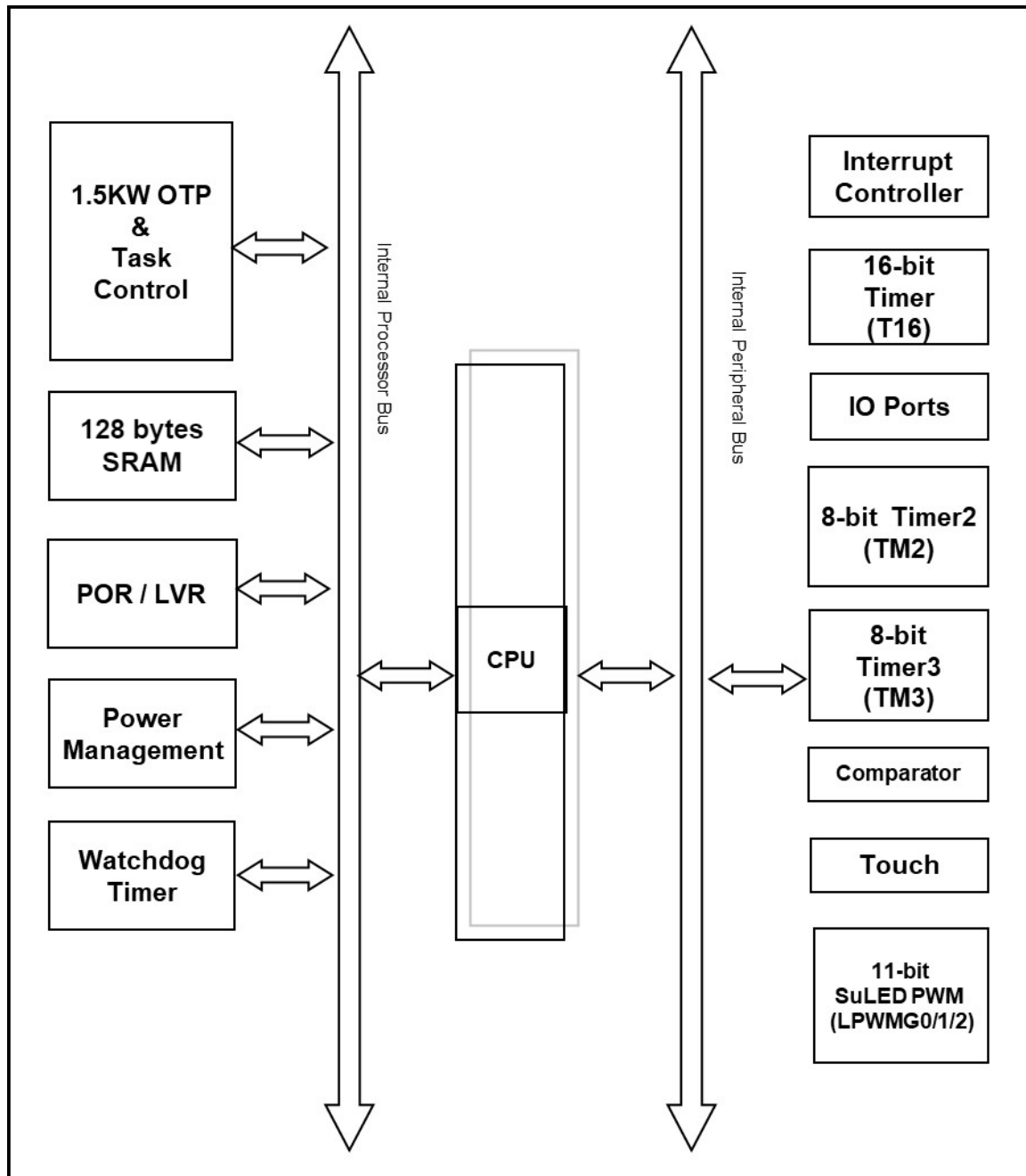
图 1: PMS160B 系统方框图
