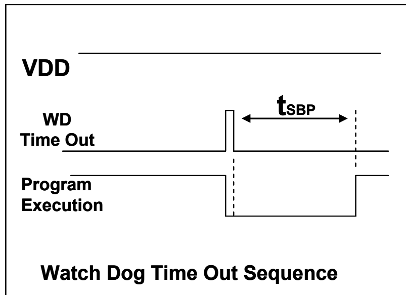
图 10: 看门狗超时溢出时序图
