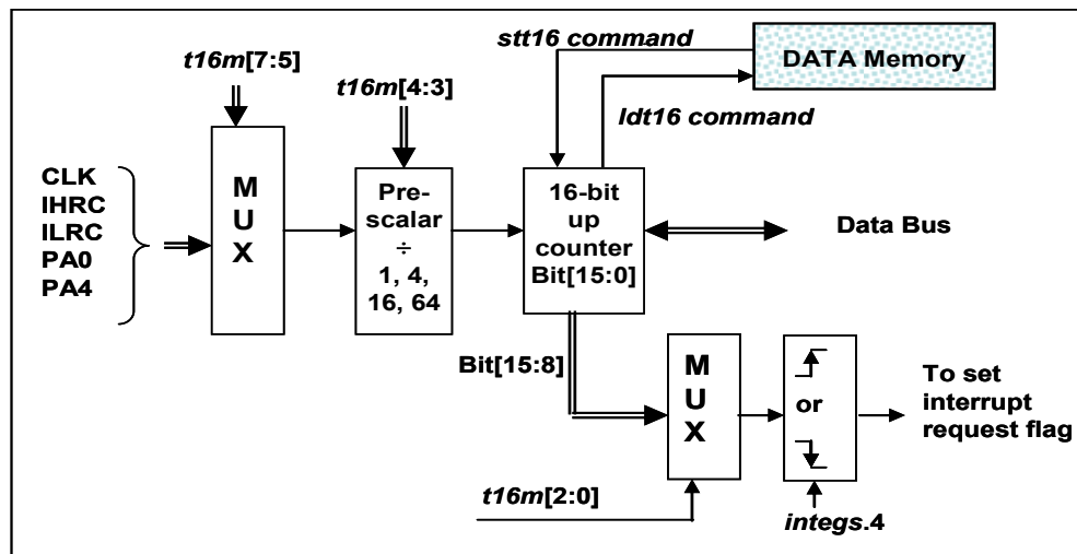
图 9: Timer16 模块框图
