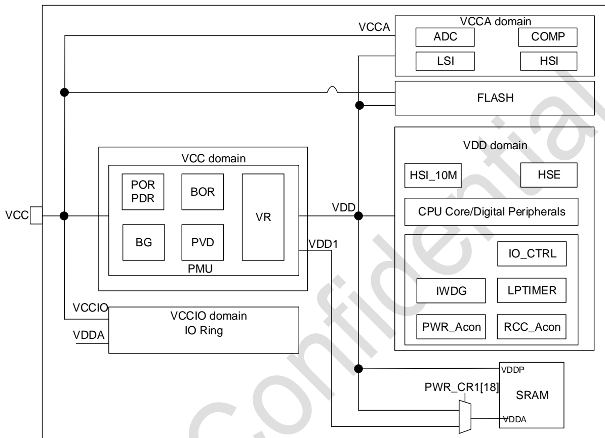
图 2-2 电源框图
