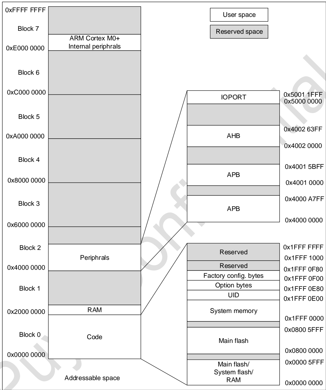
图 4-1 存储器映射
