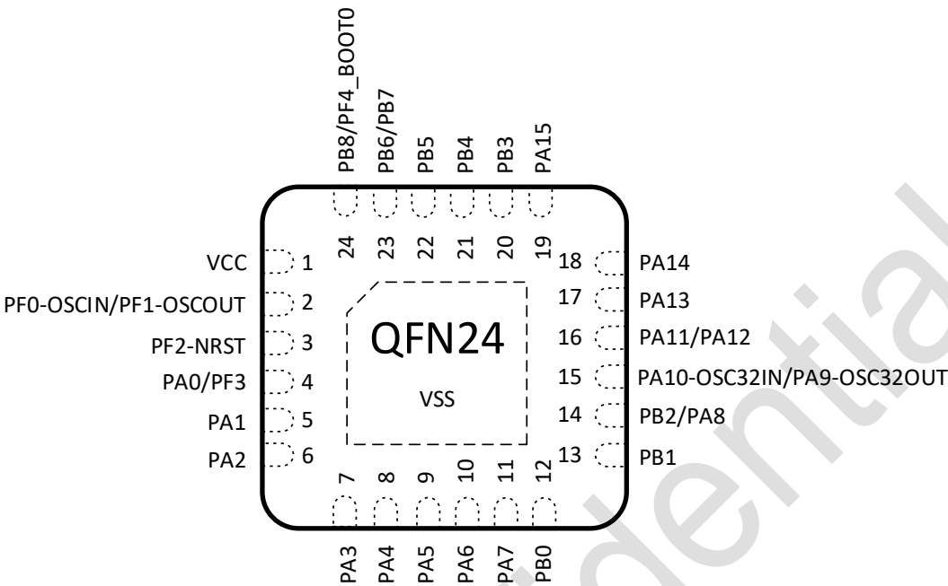
图 3-1 QFN24 Pinout1 PY32C616E1xU-E
