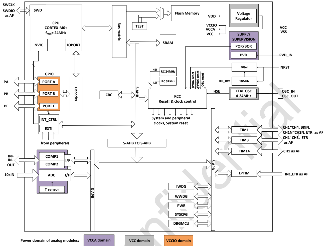
图 1-1 功能模块
