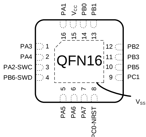
图 3-1 QFN16 Pinout1 PY32C642W15U
