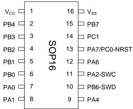
图 3-1 SOP16 Pinout1 MS32C001W12S
