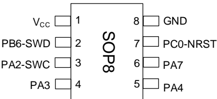
图 3-4 SOP8 Pinout1 MS32C001L12S
