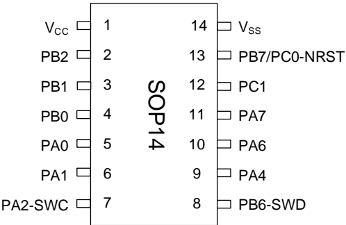
图 3-2 SOP14 Pinout1 MS32C001D12S
