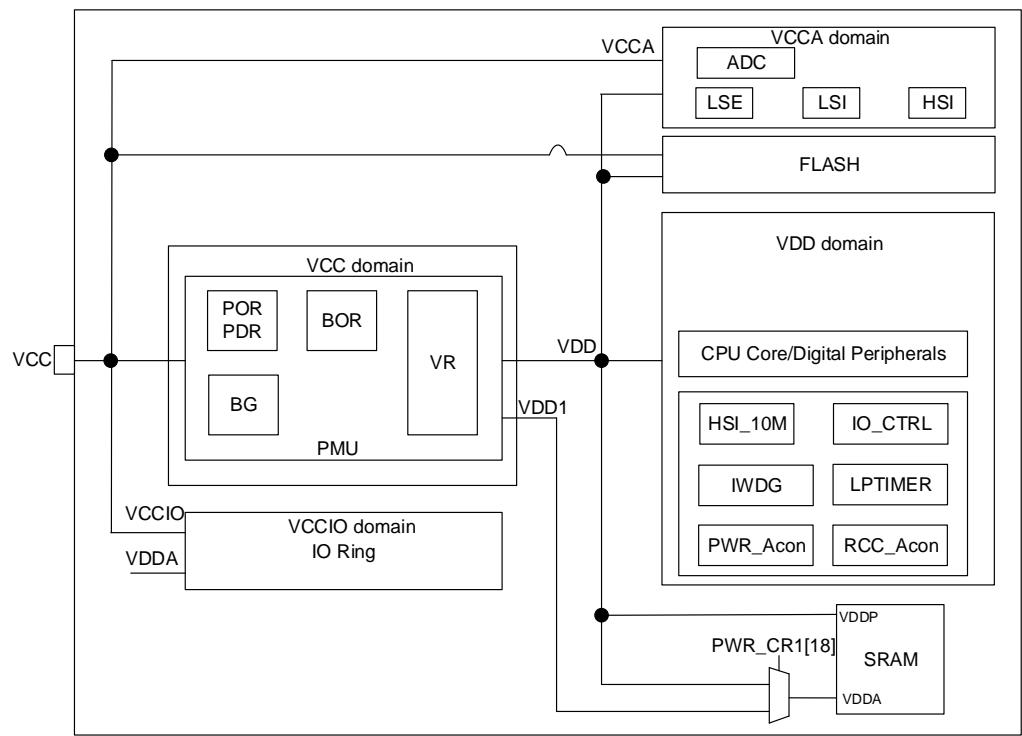
图 2-2 电源框图
