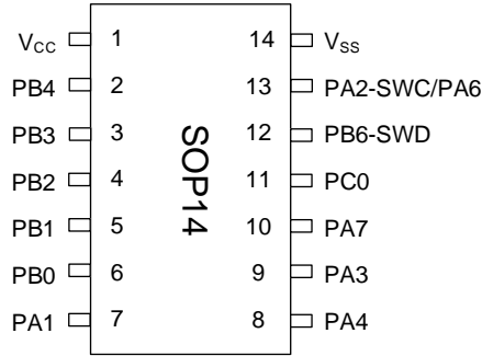
图 3-3 SOP14 Pinout2 MS32C001D22S
