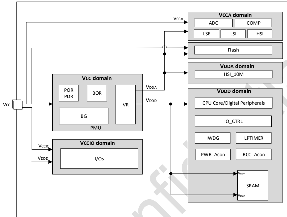
图 2-2 电源框图
