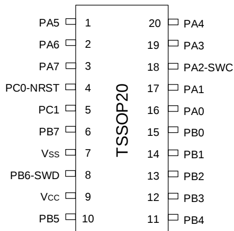
图 3-1 TSSOP20 Pinout1 MS32C001F14P6-C (Top view)
