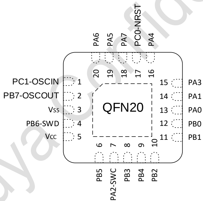
图 3-2 QFN20 Pinout1 MS32C001F14U6-C (Top view)
