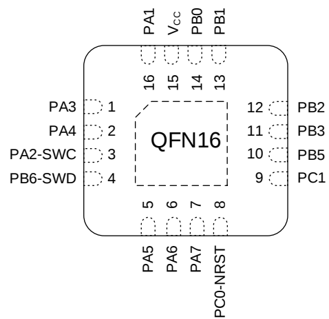
图 3-3 QFN16 Pinout1 MS32C001W14U6-C (Top view)
