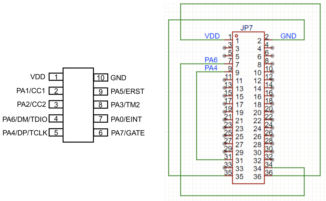
图. 9.1: P-003x 的 Jumper7 原理图
