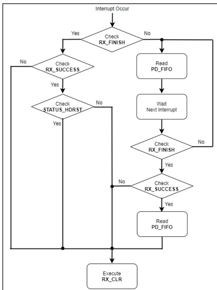
图. 5.15: RX 流程图
