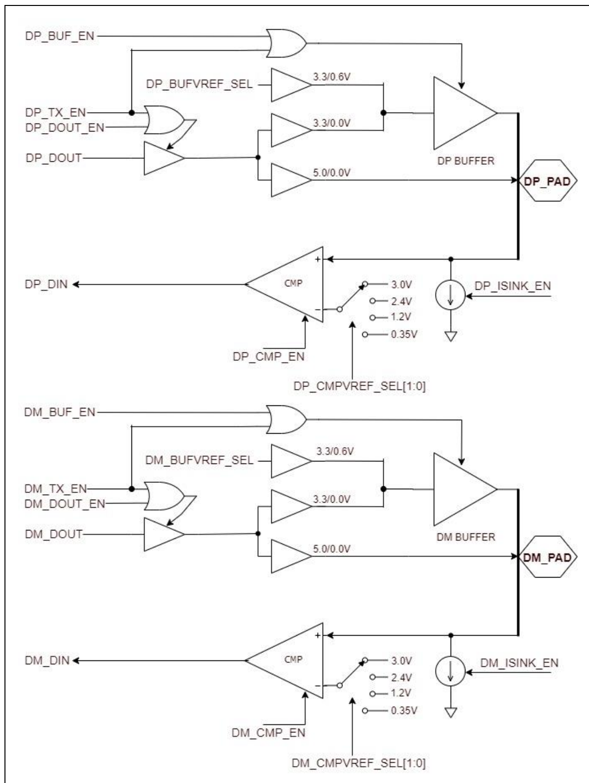
图. 5.19: DP 和 DM 硬件框图
