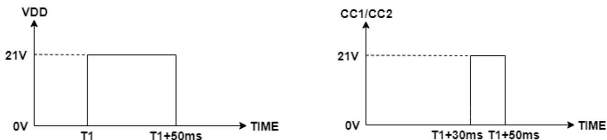
图 3.1: CC1/CC2 最大额定值测试方法
