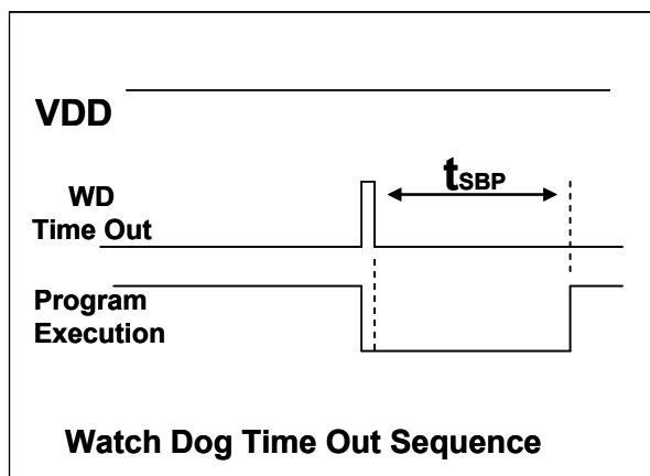
图 5.7: 看门狗超时溢出时序图
