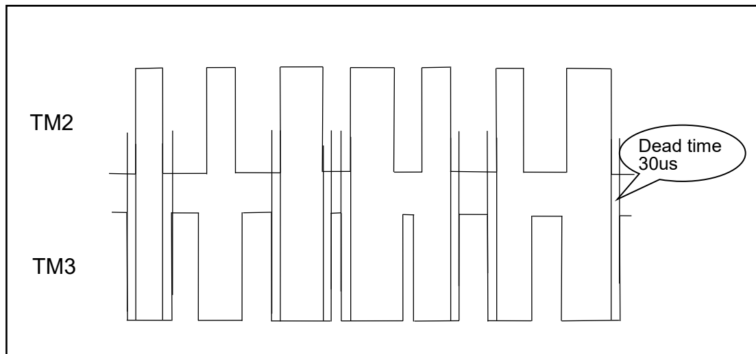
图 15： 两路互补 PWM 波形
