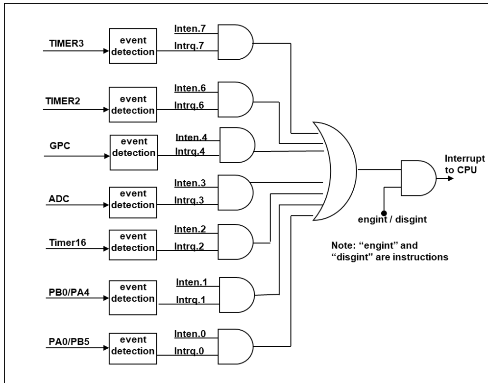
图 17：中断控制器硬件框图
