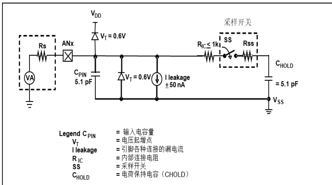
图 20：模拟输入模型
