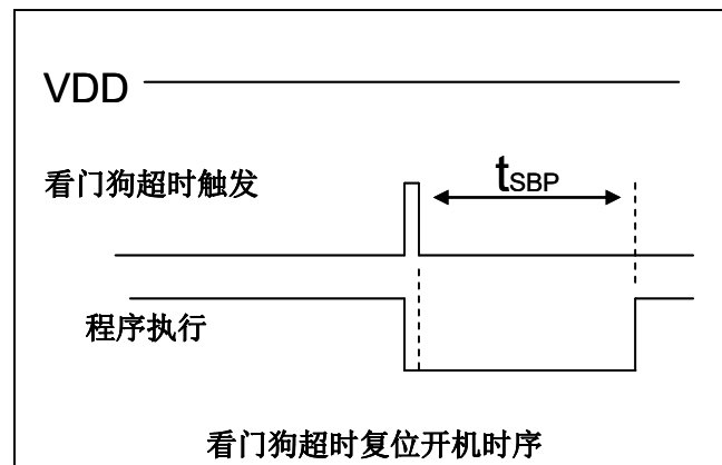
图 16：看门狗超时溢出时序图
