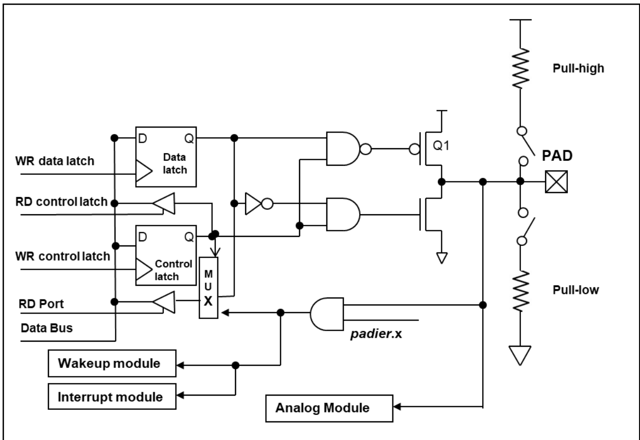
图 18: IO 引脚缓冲区硬件图
