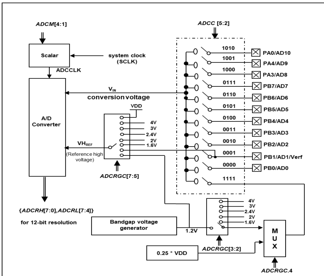
图 19: ADC 模块框图
