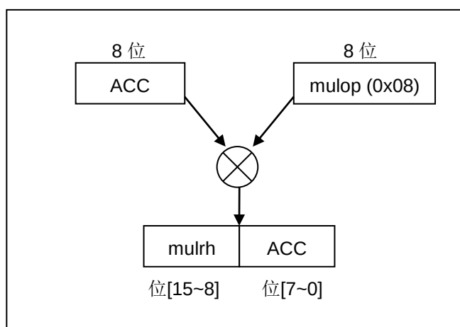
图 23：硬件乘法器框图
