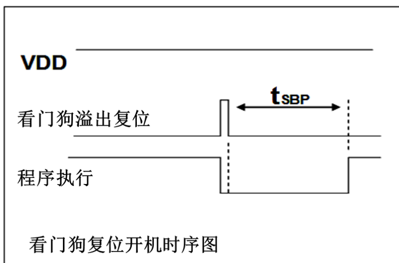
图 18：看门狗超时溢出时序图
