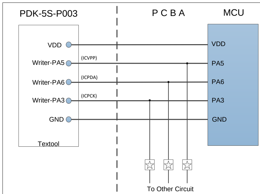
图 24：在板烧录示意图
