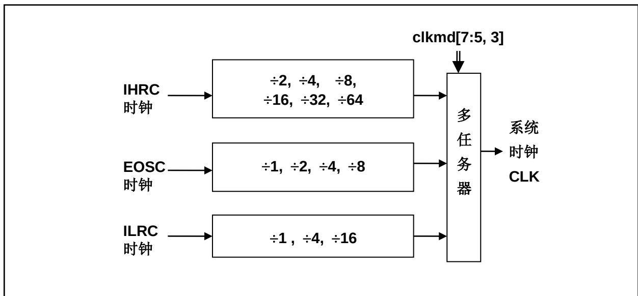
图 3：系统时钟源选项
