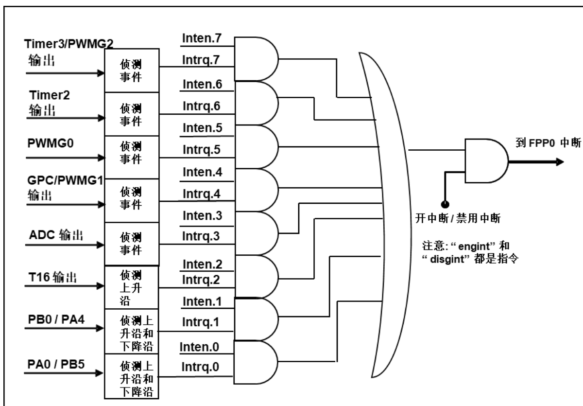
图 18：中断控制器硬件框图
