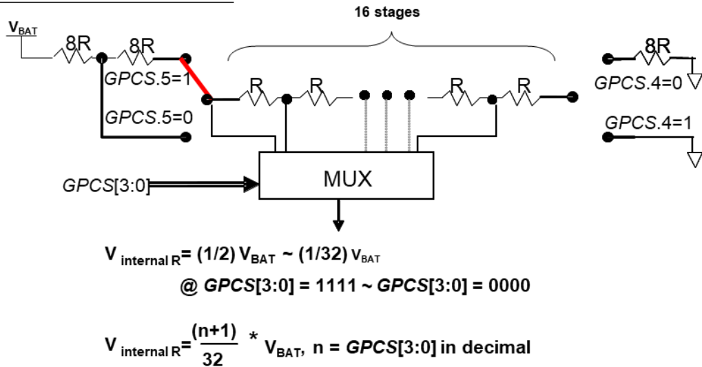
图 8: V_{internal\ R} 硬件接法( GPCS.5=1 & GPCS.4=1 )
