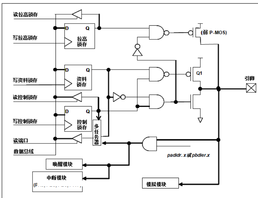
图 19: IO 引脚缓冲区硬件图
