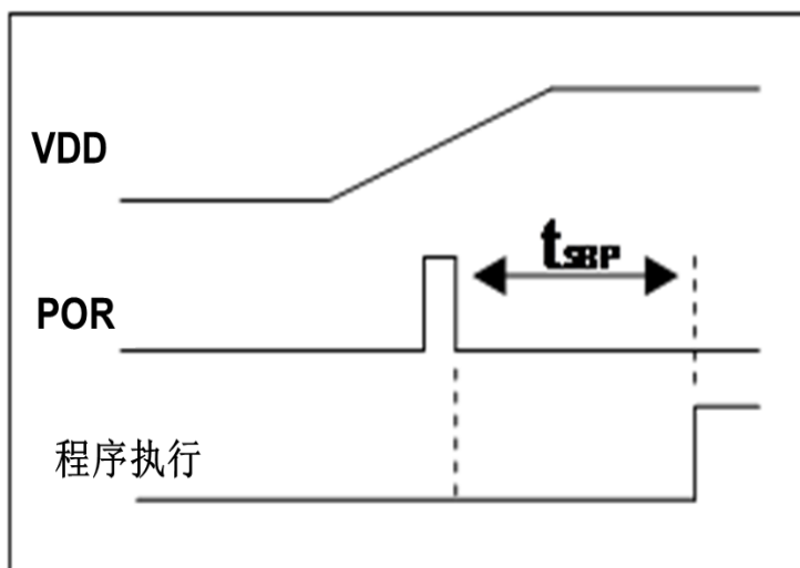
图 1：上电复位时序
