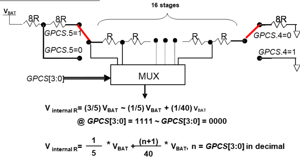
图 7: V_{internal\ R} 硬件接法( GPCS.5=1 & GPCS.4=0 )
