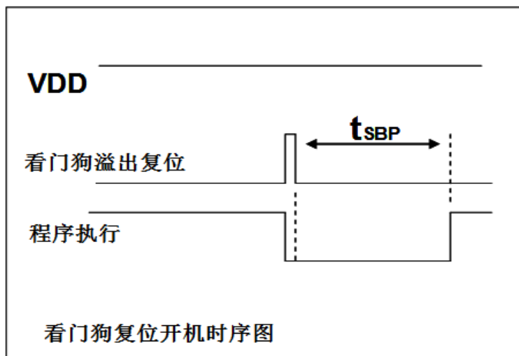
图 17：看门狗超时溢出时序图
