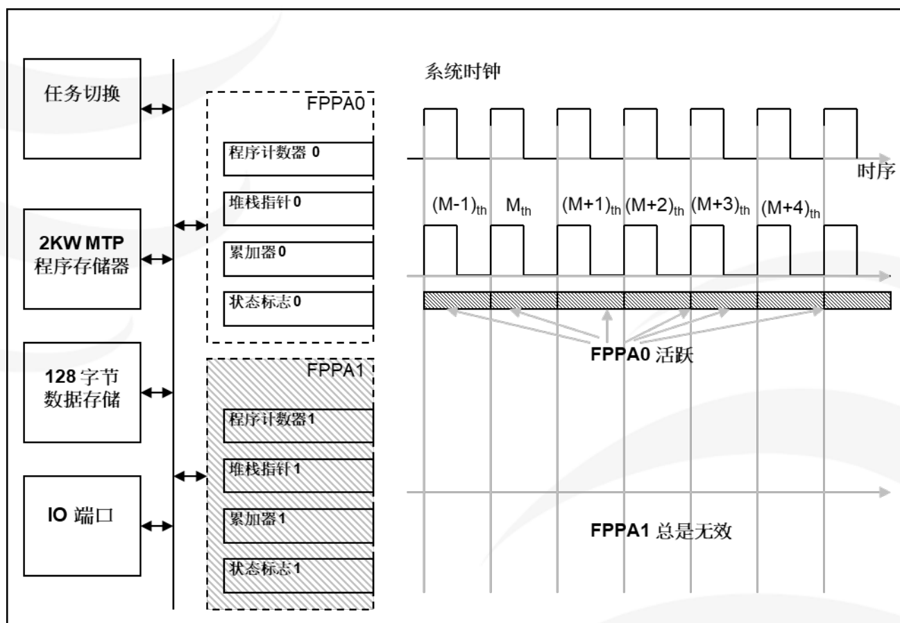
图 2：一个处理单元工作模式下的时序
